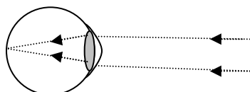
รูป ข .ภาพชัดที่จุดไกล
