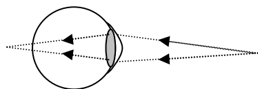
รูป ก.จุดใกล้ภาพไม่ชัด
