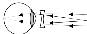
รูป ค .การแก้ไขใช้เลนส์เว้า
