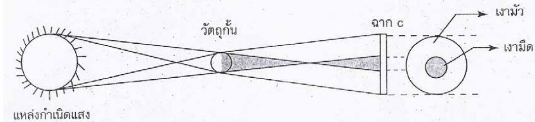
3.3 วางฉากอยู่ที่จุด C จะเกิดเงามืดอย่างเดียวยอยู่บนฉากกัน
