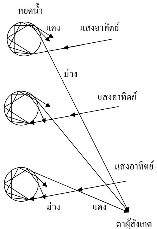
รูป 3 ข รุ้งทุติยภูมิ
