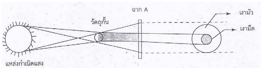
3.1 วางฉากอยู่ที่จุด A จะเกิดเงามัวล้อมรอบเงามืดอยู่บนฉากกัน
