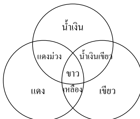
รูป แสดงการผสมแสงสีปฐมภูมิบนฉากขาว
