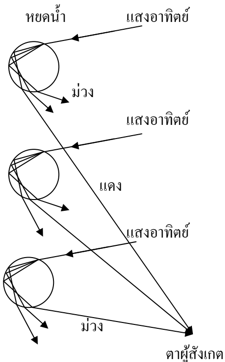
รูป 3 ก รุ้งปฐมภูมิ
